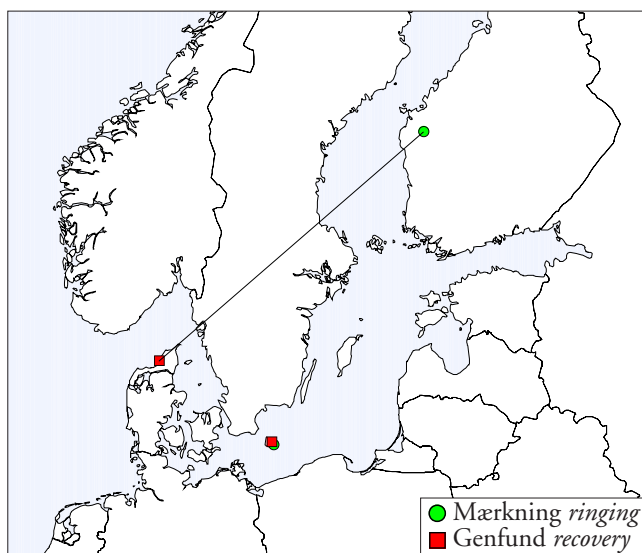
Fig. 1. Mærkningslokaliteter forbundet til genfundlokaliteter for perleugle genfundet i Danmark (n=2). Ringing locations connected to recovery sites of tengmalm's owl recovered in Denmark (n=2).
